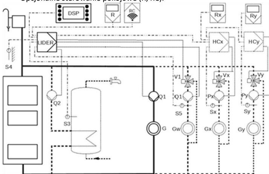
Schemat połączeń:
