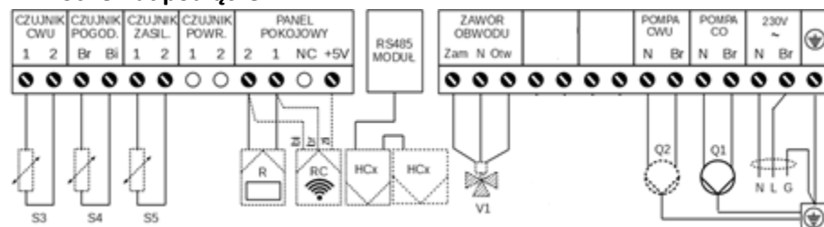
Schemat połączeń:
